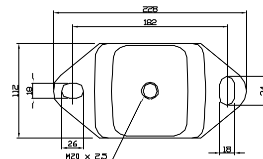
BAKRE GUMMIDEMPER
