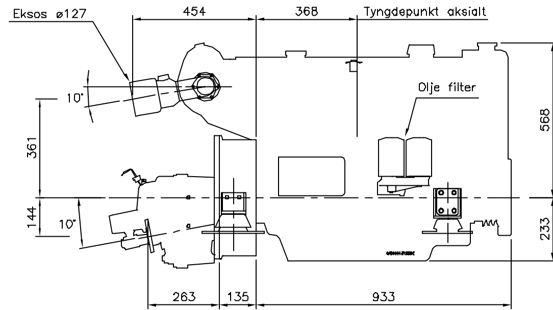
HØYRE SIDE
