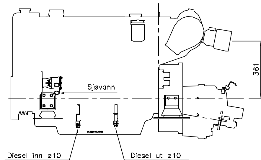
VENSTRE SIDE
