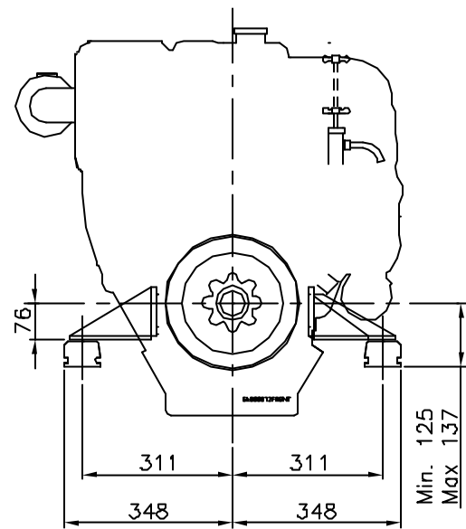
FORFRA
