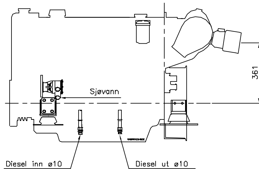
VENSTRE SIDE
