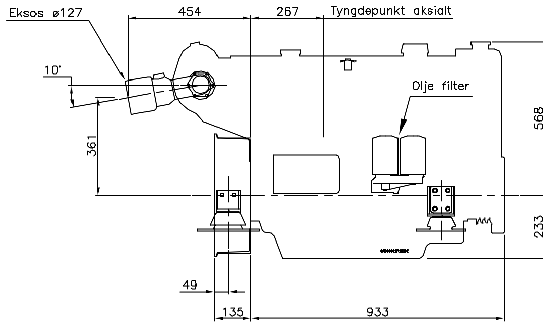
HØYRE SIDE
